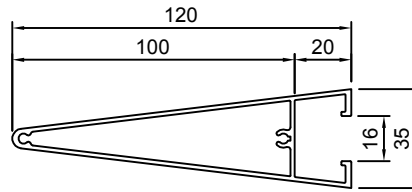
YN-HI325 단중: 1.262 kg/m 외주위장: 352.0 mm
