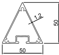
KU-018-2 0.679KG/M
