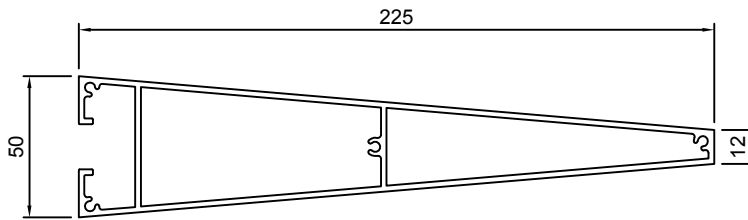
YN-KS-027A 단중: 3.190 kg/m 외주위장: 630.9 mm
