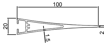
KU-053-1 0.982KG/M
