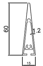
KU-107A 0.594KG/M
