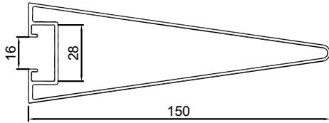
TKS-081 단중: 1.569kg/m 외주위장: 419.7mm
