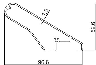
KU-144C 1.076KG/M
