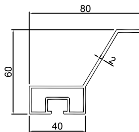
KU-279 0.914KG/M
