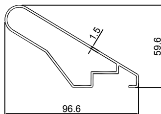
KU-144A 0.999KG/M
