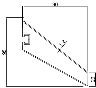
KU-561A 1.068KG/M
