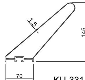
KU-331 2.342
