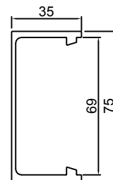
KU-489-3 ???: 1.041kg/m ?????: 295 mm
