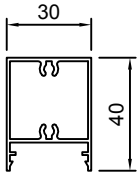
YN-HI263 단중: 0.548 kg/m 외주위장: 170.5 mm
