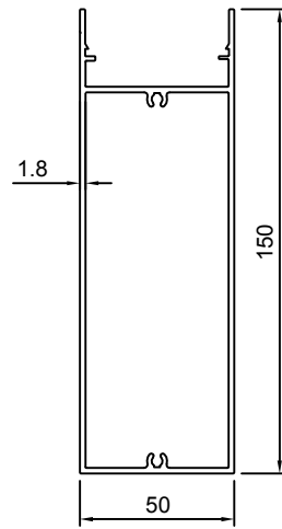
YN-HI389 단중: 2.019 kg/m 외주위장: 463.5 mm
