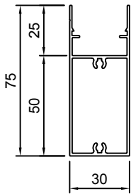
YN-HI385 단중: 0.832 kg/m 외주위장: 275.3 mm
