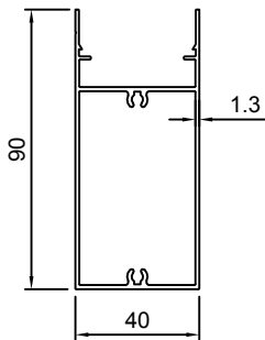
YN-HI391 단중: 1.008 kg/m 외주위장: 325.5 mm
