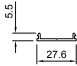
YN-HI264 단중: 0.137 kg/m 외주위장: 76.3 mm
