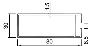
KU-275B 0.978KG/M
