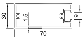
FJ-007 0.980 kg/m 225.9
