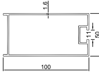
KU-276 1.417KG/M
