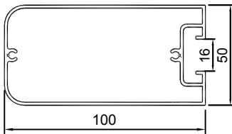
TKS-062-1 1.41 kg/m 347.6
