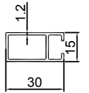
KU-206-1 0.298KG/M
