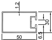
KU-303 0.598KG/M
