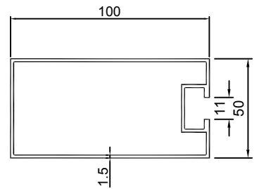
KU-204 1.36KG/M
