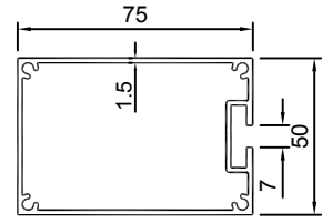
KU-130-1 1.21KG/M
