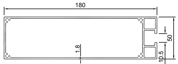
KU-209 2.638KG/M
